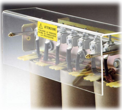
Protezioni morsettiere
